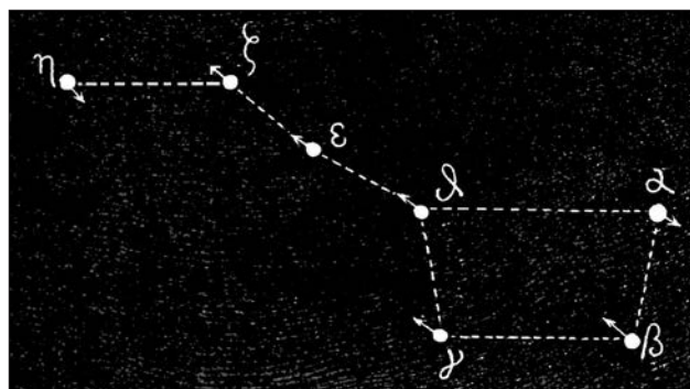
Fig. 5 : Mouvement des étoiles de la Grande Ourse.
