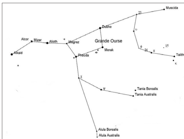
Fig. 3 : étoiles de la Grande Ourse.
