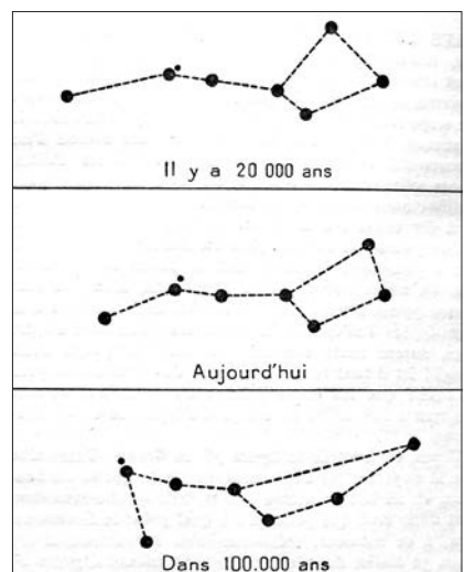
Fig. 6 : déplacement des étoiles de la Grande Ourse.
